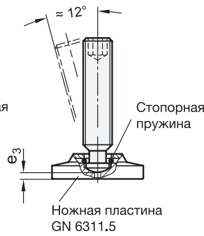
Примеры сборки
